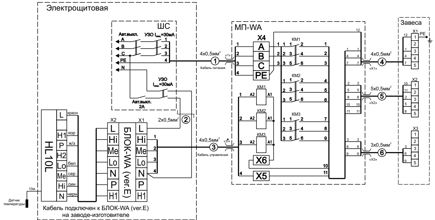
Рисунок 3. Схема подключения БЛОК-WA (ver.E) к модулю МП-WA одной завесы
