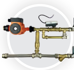
Узел смешения УСН-6
